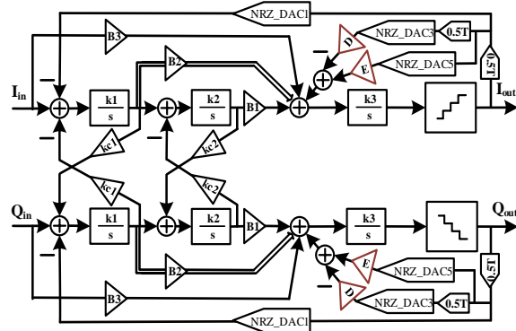
شکل ۱۲: ساختار مدولاتور متعامد پیشنهادی پس از تلفیق دو DAC
