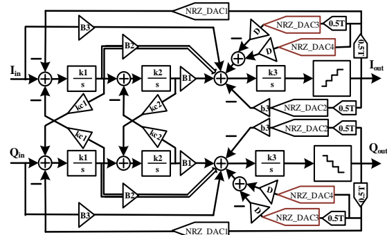
شکل ۱۱: ساختار مدولاتور متعامد پس پیاده سازی RZ-DAC به وسیله دو NRZ-DAC
