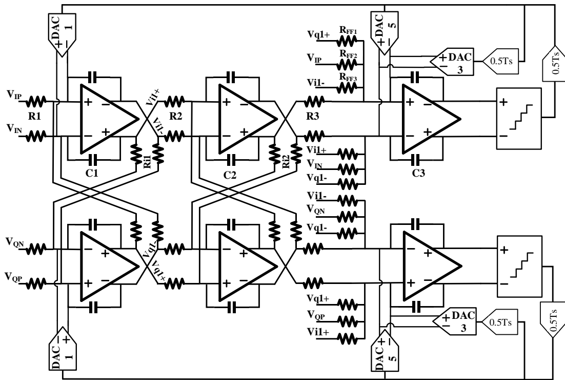
شکل ۱۴: شکل مداری مدولاتور طراحی شده
