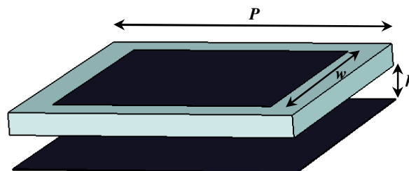
شکل ۲: نمای کلی سلول واحد مربعی و پچ مربعی روی آن. تغییر پارامترهای w و h موجب تغییر در فاز بازگشتی هر سلول واحد می شود.
