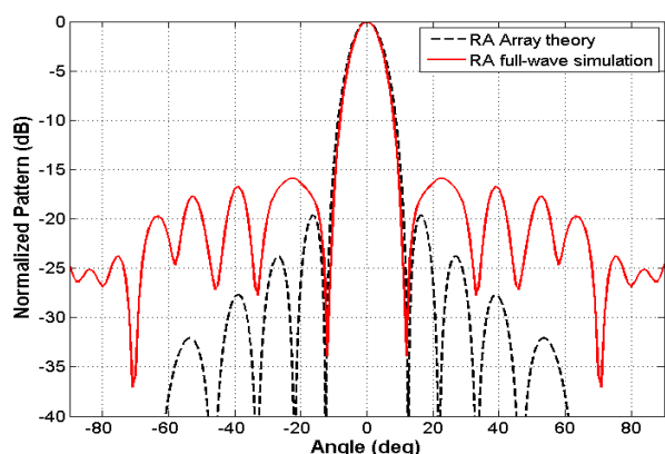
شکل ۱۱: مقایسه الگوی میدانی دور آنتن آرایه انعکاسی حاصل از روش عددی تئوری آرایه‌ها با نتایج شبیه‌سازی تمام موج.
