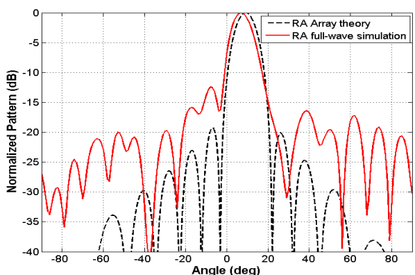
شکل ۱۲: مقایسه الگوی میدانی دور آنتن آرایه انعکاسی حاصل از روش تئوری آرایه‌ها با نتایج شبیه‌سازی تمام موج، در حالتی که زمین ساختار در حدود 0.5^\circ چرخیده است.
