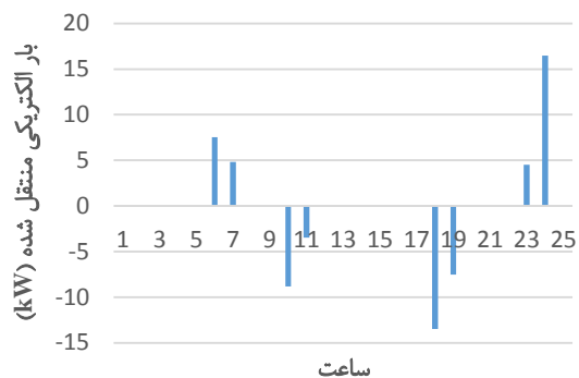
شکل ۵: تغییرات بار الکتریکی ناشی از برنامه پاسخ تقاضا (مطالعه اول)
