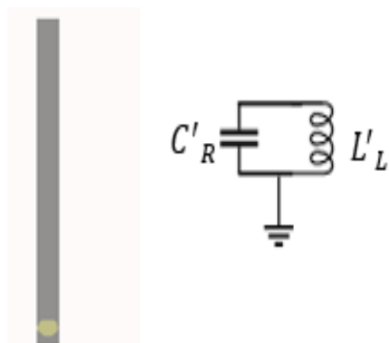
شکل ۵: ساختار و مدار معادل استاب اتصال کوتاه
