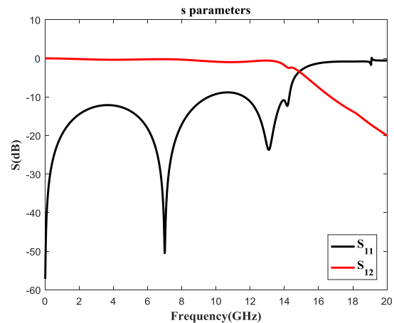
شکل ۴: نتایج شبیه‌سازی سلول خط تأخیر پهن باند
