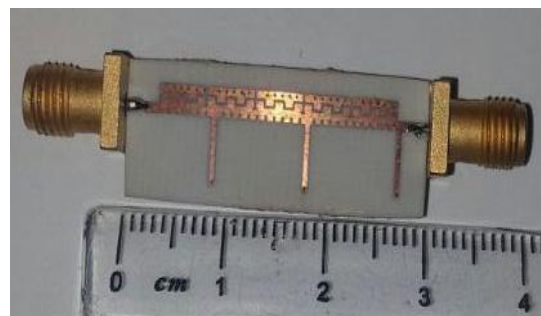
شکل ۱۲: فیلتر فوق پهن باند ساخته شده
