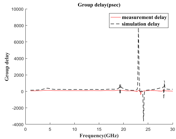
شکل ۱۵: مقدار تأخیر گروه فیلتر فوق پهن باند پیشنهادی
