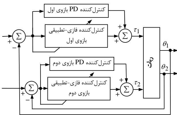
شکل (۱): بلوک دیاگرام کنترل کننده فازی- تطبیقی
