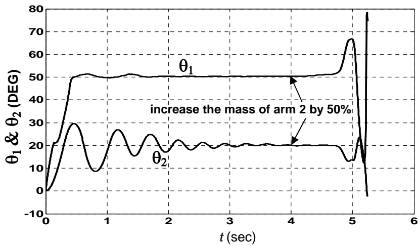
شکل (۱۲): مسیر بازوهای اول و دوم ربات با کنترل کننده فازی- ممدانی با افزایش جرم بازوی دوم به اندازه ۵۰ درصد مقدار اولیه در ثانیه ۴ (سیستم ناپایدار شده است)
