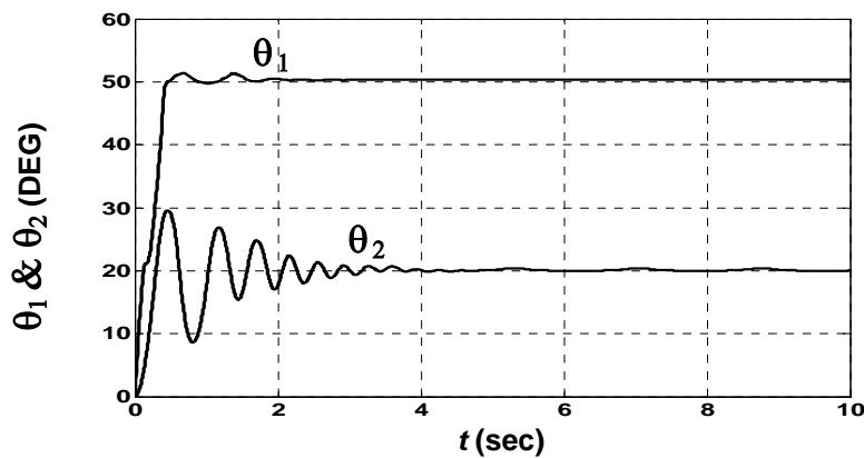
شکل (۶): مسیر بازوهای اول و دوم ربات با کنترل کننده فازی-ممدانی
