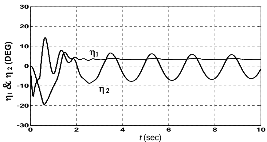
شکل (۹): ارتعاش بازوهای اول و دوم ربات با کنترل کننده فازی-ممدانی
