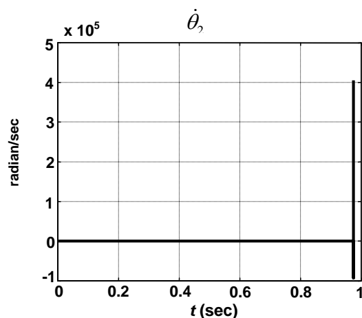
شکل (۱۶): سرعت زاویه بازوی دوم در نقطه تکین \theta_2 = 180^\circ
