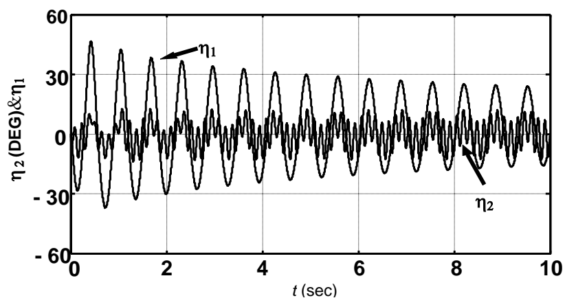
شکل (۱۰): ارتعاش بازوهای اول و دوم ربات با کنترل کننده گشتاور محاسباتی
