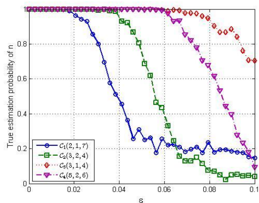
شکل ۸: احتمال تخمین صحیح پارامتر n بر حسب نرخ خطای کانال
