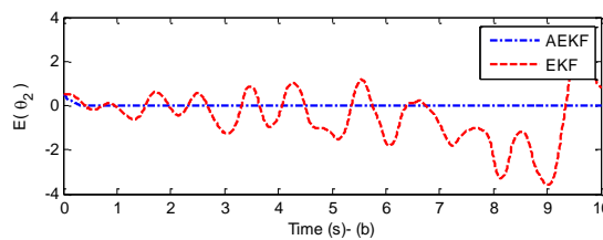
شکل ۵: تخمین حالت های ربات دو درجه آزادی؛ (a) مکان لینک دوم، (b) خطای تخمین مکان لینک دوم
