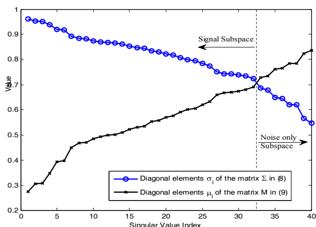
شکل ۶: نمونه ای از عناصر قطری \sigma_i و \mu_i ، به ترتیب، مربوط به ماتریس‌های \Sigma و M ، حاصل از معادلات (۸) و (۹) برای یک فریم سیگنال گفتار نوعی با
