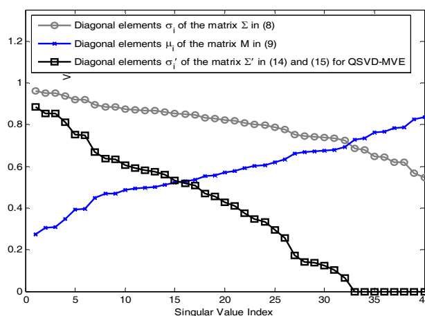
شکل ۷: نمونه‌ای از عناصر قطری \sigma_i ، \mu_i و \sigma'_i ، به ترتیب، مربوط به ماتریس‌های \Sigma ، M و \Sigma' در الگوریتم QSVD-MVE، حاصل از معادلات (۸)، (۹) و (۱۵) برای یک فریم سیگنال گفتار با N = 40
