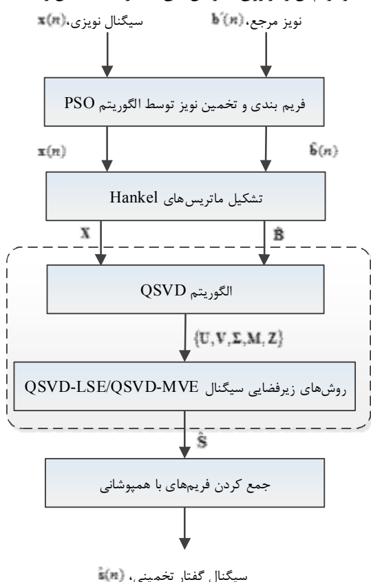
شکل ۴: فرآیند الگوریتم‌های بهبود کیفیت گفتار مبتنی بر QSVD (PCQSVD-LSE-PSO و PCQSVD-MVE-PSO).
