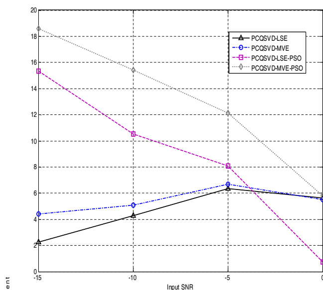
شکل ۱۰: میانگین میزان بهبود سیگنال به نویز با به کارگیری الگوریتم‌های PCQSVD-LSE، PCQSVD-MVE، PCQSVD-LSE-PSO و PCQSVD-MVE-PSO با چهار نوع نویز مختلف.
