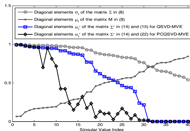
شکل ۸: عناصر قطری \sigma_i ، \mu_i و \sigma'_i مربوط به ماتریس‌های \Sigma ، M و \Sigma' در الگوریتم‌های QSV-D-MVE و PCQSV-D-MVE، حاصل از معادلات (۸)، (۹)، (۱۵) و (۲۲) برای یک فریم از سیگنال گفتار با N = 40 .
