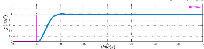
شکل ۲۱: زاویه پیشروی هواپیمای بدون سرنشین به روش BTT با کنترل‌کننده Backstepping
