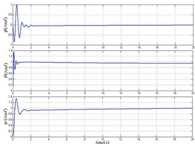
شکل ۱۸: رفتار زوایای Roll، Pitch و Yaw با کنترل‌کننده Backstepping
