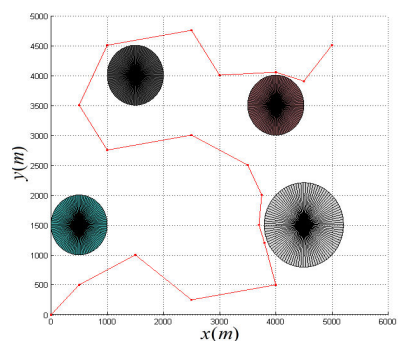
شکل ۱۵: مسیر اصلاح‌شده برای احتراز از موانع، نمای صفحه xy
