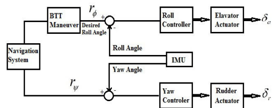
شکل ۷: بلوک دیاگرام هدایت هواپیما به روش BTT [۱۴]
