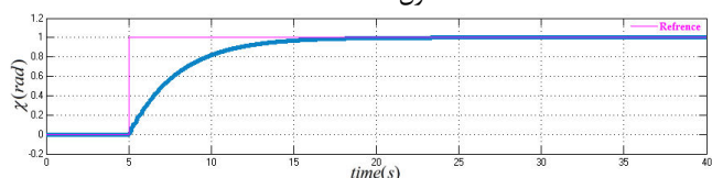
شکل ۲۳: زاویه پیشروی هواپیمای بدون سرنشین به روش BTT با کنترل‌کننده Backstepping+SMC
