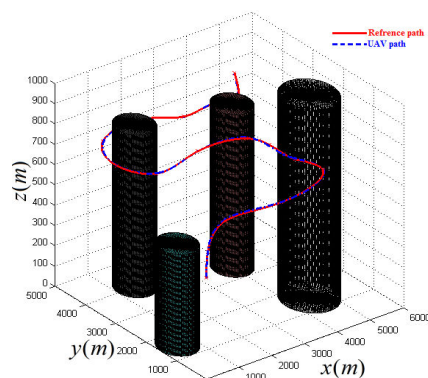
شکل ۲۹: دنبال کردن مسیر تولیدشده UAV به روش BTT و کنترل‌کننده
