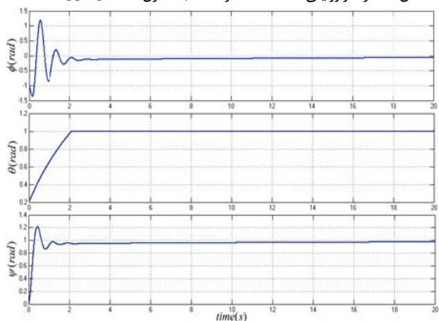
شکل ۱۹: رفتار زوایای Roll، Pitch و Yaw با کنترل‌کننده SMC
