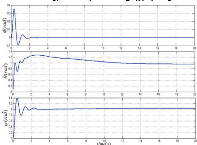
شکل ۲۰: رفتار زوایای Roll، Pitch و Yaw با کنترل‌کننده SMC
