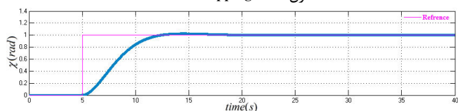
شکل ۲۲: زاویه پیشروی هواپیمای بدون سرنشین به روش BTT با کنترل‌کننده SMC
