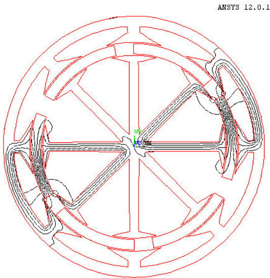
شکل ۳: موتور سوئیچ رلوکتانس دارای دو استاتور و نمایش خطوط شار [۱۴]
