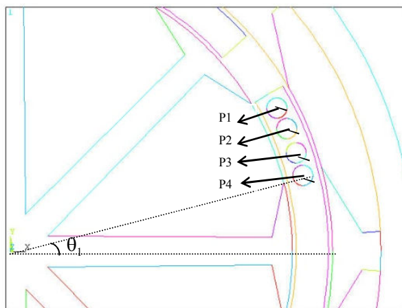
شکل ۴: متغیرهای در نظر گرفته‌شده به‌منظور بهینه‌سازی موتور سوئیچ رلوکتانس دارای دو استاتور
