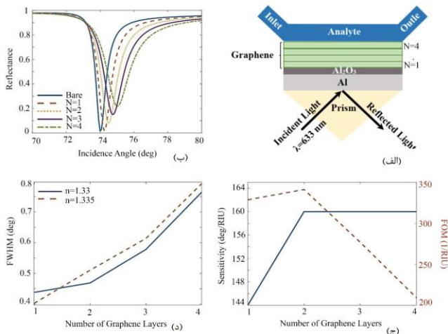
شکل ۳- (الف) شماتیک ساختار حسگر با ۴ لایه گرافن، (ب) حداقل بازتاب برای ۵ حالت (بدون گرافن و با ۴ لایه گرافن)، (ج) حساسیت و FOM برای تعداد لایه‌های مختلف گرافن، (د) FWHM به‌ازای تعداد لایه‌های مختلف گرافن و ضرایب شکست آنالیت 1/335 و 1/335 .
