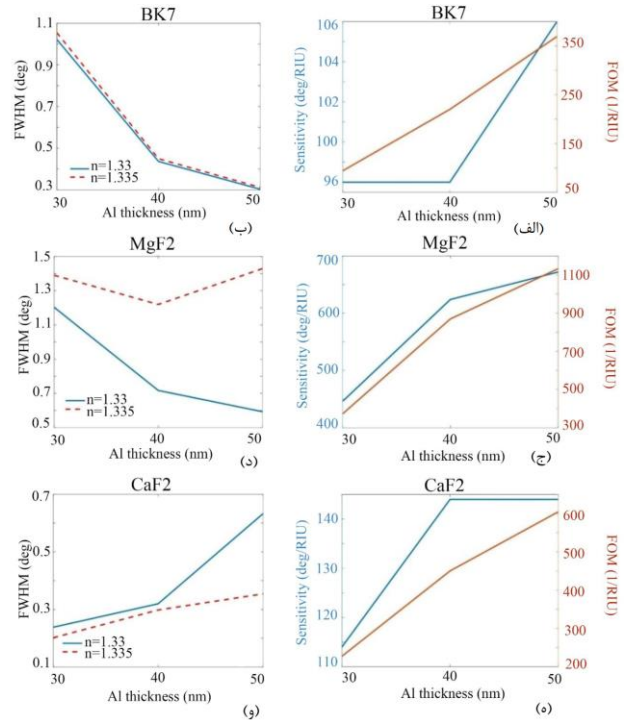
شکل ۲- حساسیت، FWHM و ساختار برای منشورهای به ترتیب (الف، ب) \text{BK}_7 ، (ج، د) \text{MgF}_2 و (ه، و) \text{CaF}_2 .
