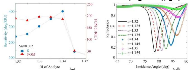
شکل ۸- بررسی عملکرد ساختار نهایی به‌ازای تغییرات ضریب شکست آنالیت n_i = 1/355 - 1/33 ، (الف) حداقل بازتاب به همراه (ب)
