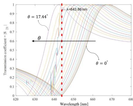
شکل ۳- طیف‌های انتقال شبیه‌سازی شده برای فراسطح مشتق‌گیر مکانی مرتبه دوم (\frac{a^2}{\alpha^2} f(x, y)) ، تحت تابش نور با قطبش y - و در صفحه \varphi = 0^\circ به ازای زوایای مختلف \theta نسبت به راستای عمودی به دست آمده است. خط چین قرمز طول موج عملیاتی (\lambda = 643.86 \text{ nm}) را نشان می‌دهد.
