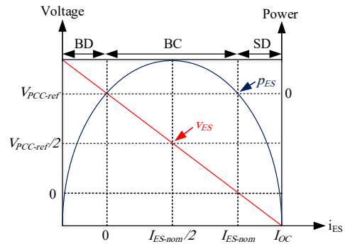
شکل ۲- منحنی ولتاژ و توان فنر DC سری در نواحی عملکرد مختلف [۱۷]
