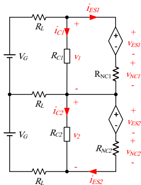
شکل ۶- مدار معادل فنر DC سری در ریزشبه DC دوقطبی [۱۵]
