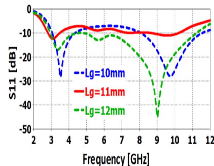
شکل ۸- تغییرات S_{11} برای تغییرات صفحه زمین
