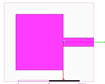
شکل ۲ - طرح دوم آنتن پیشنهادی
