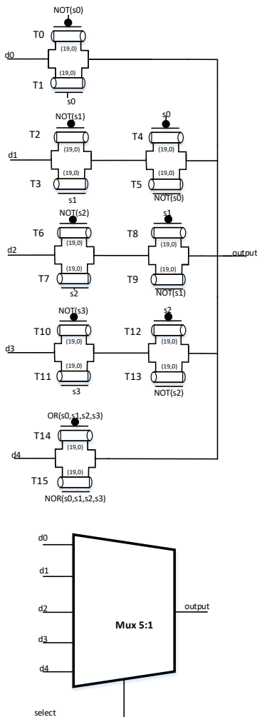
شکل ۴- شماتیک مدار مالتی پلکسر ۵×۱
