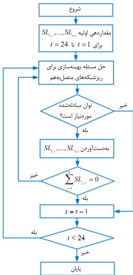
شکل ۲: روندنمای روش پیشنهادی برای مدیریت توزیع شده ریز شبکه‌های متصل به هم
