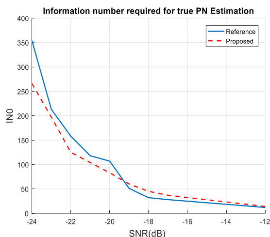
شکل ۹: تعداد نمونه‌های اطلاعات موردنیاز برای تخمین صحیح دنباله PN
