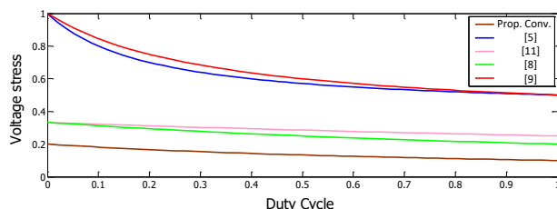
شکل ۷: مقایسه تنش ولتاژ بر روی کلیدهای فعال مبدل پیشنهادی و کلیدهای فعال برخی از مبدل‌های دیگر
