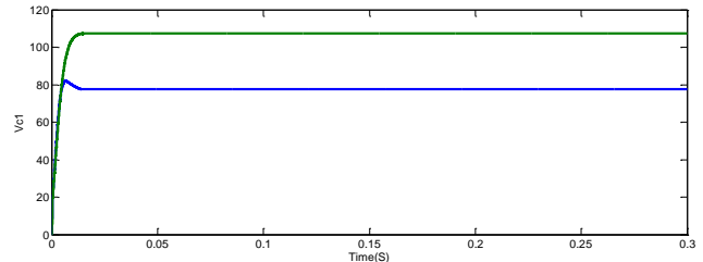
شکل ۱۷: ولتاژ خازن C_1 در حالت CCM
