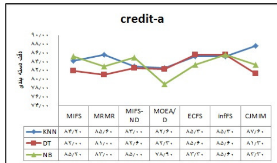
شکل ۷: دقت دسته‌بندی KNN، DT و NB به ازای k=6
