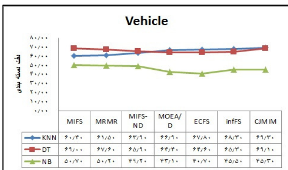
شکل ۵: دقت دسته‌بندی KNN، DT و NB به ازای k=۱۰
