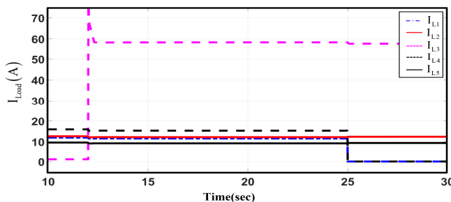
شکل ۸: جریان لحظه‌ای بارهای ریزشبه‌های dc
