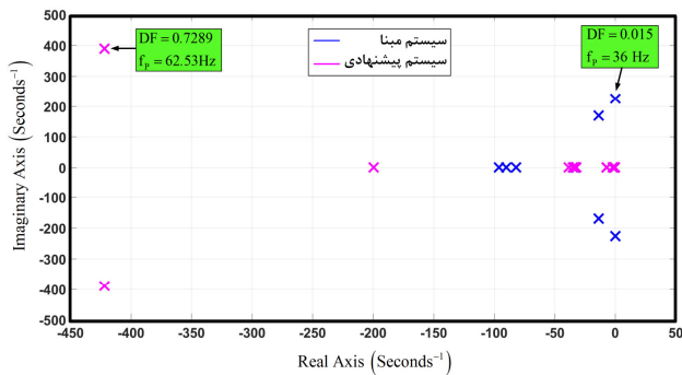
شکل ۷: مدهای غالب فرکانس پایین ریزشبه dc برای هر دو مورد سیستم مینا و سیستم پیشنهادی
