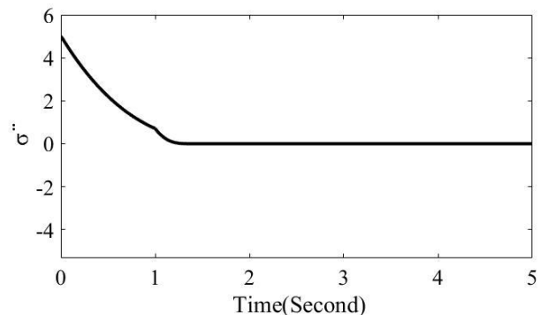
شکل ۵: نمودار همگرایی سطح لغزش مرتبه سوم ( \ddot{\sigma} )
