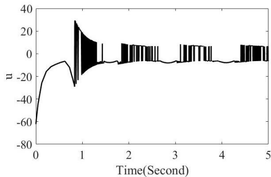
شکل ۹: نمودار ورودی کنترل بر اساس روش کنترل مد لغزشی متداول
