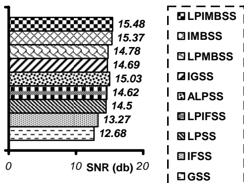
شکل (۱۰): مقایسه SNR خروجی روش‌های پیشنهادی (LPIMBSS, LPMBSS, ALPSS, LPIFSS, LPSS) و روش‌های موجود (IMBSS, IGSS, IFSS, GSS)
