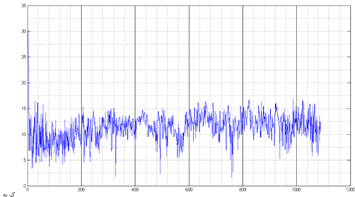
شکل ۵: نمودار حاصل از اعمال الگوریتم پیشنهادی بر روی تصویر رایس با اندازه ۳۲ در ۳۲ و تابع هزینه‌ای با 10^{-24} بردار ویژه؛ محور افقی: بردار ویژه شماره‌گذاری شده بر حسب اندازه مقدار ویژه متناظر آن (از کوچک بزرگ)، محور عمودی: معیار MF_i به ازای هر بردار ویژه
